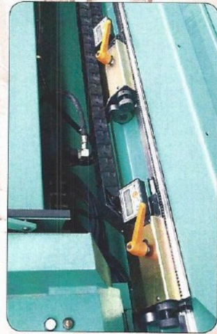
Butée à réglage rapide avec lecture sur bande magnétique.
