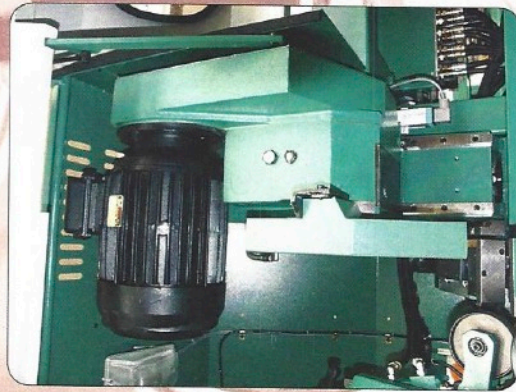
Tête de coupe à descente verticale avec angle de pénétration constant.
